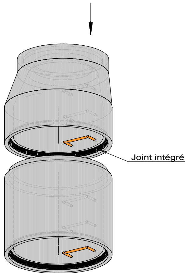
Exemple d'emboîtement d'un élément intermédiaire et cône de réduction
